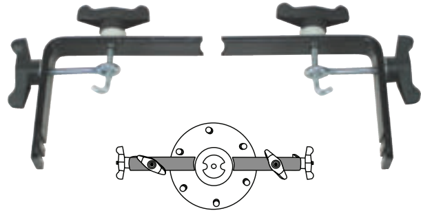
2007 SILVERADO HUB
