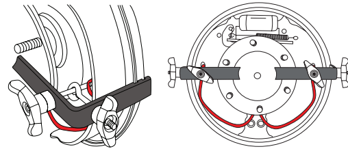
2007 SILVERADO HUB
